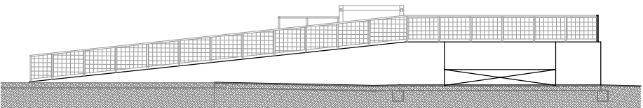
PROSPETTO NORD - OVEST scala 1:200
