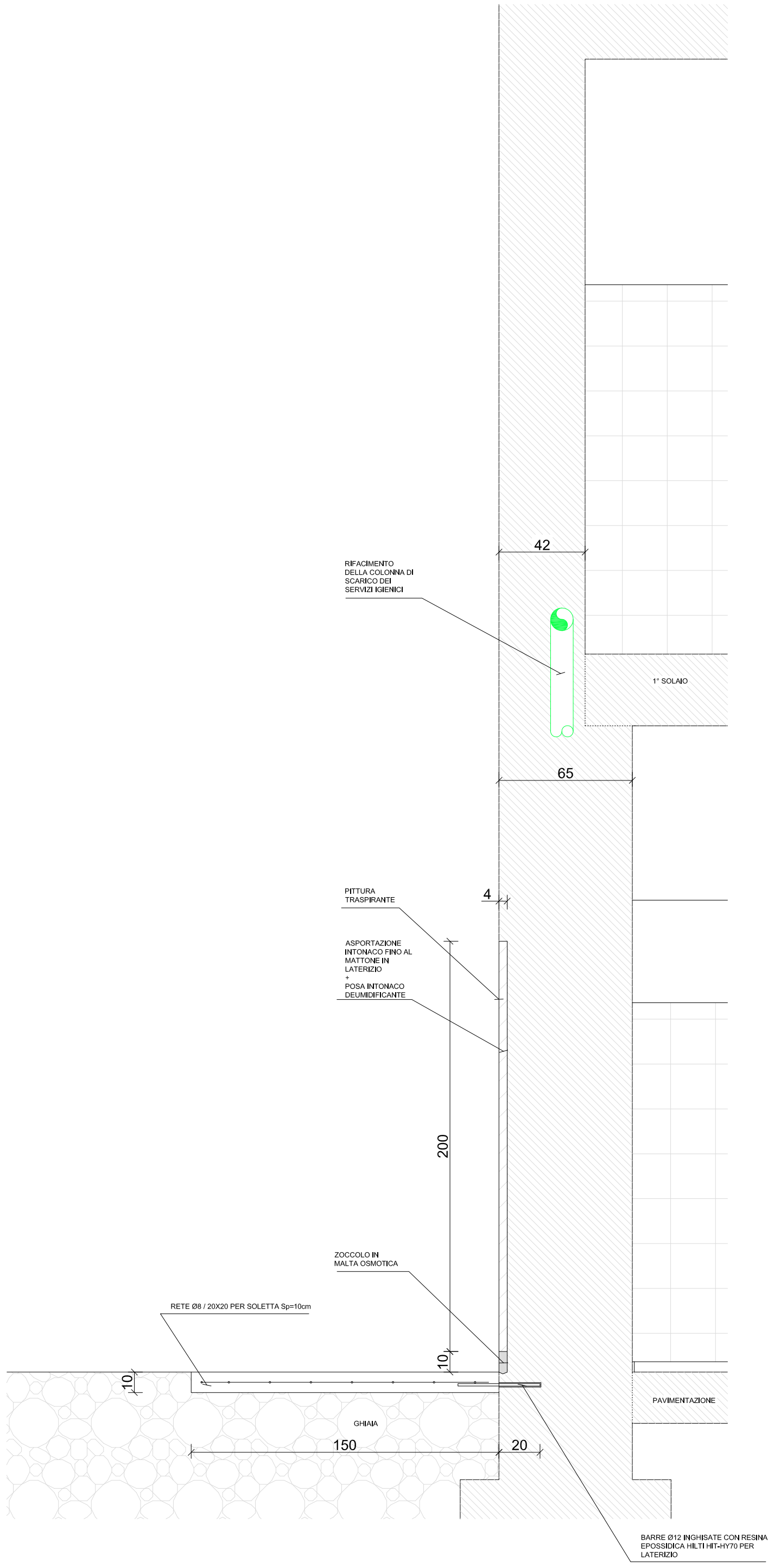
DETTAGLIO RISANAMENTO MURATURA SCALA 1:20
