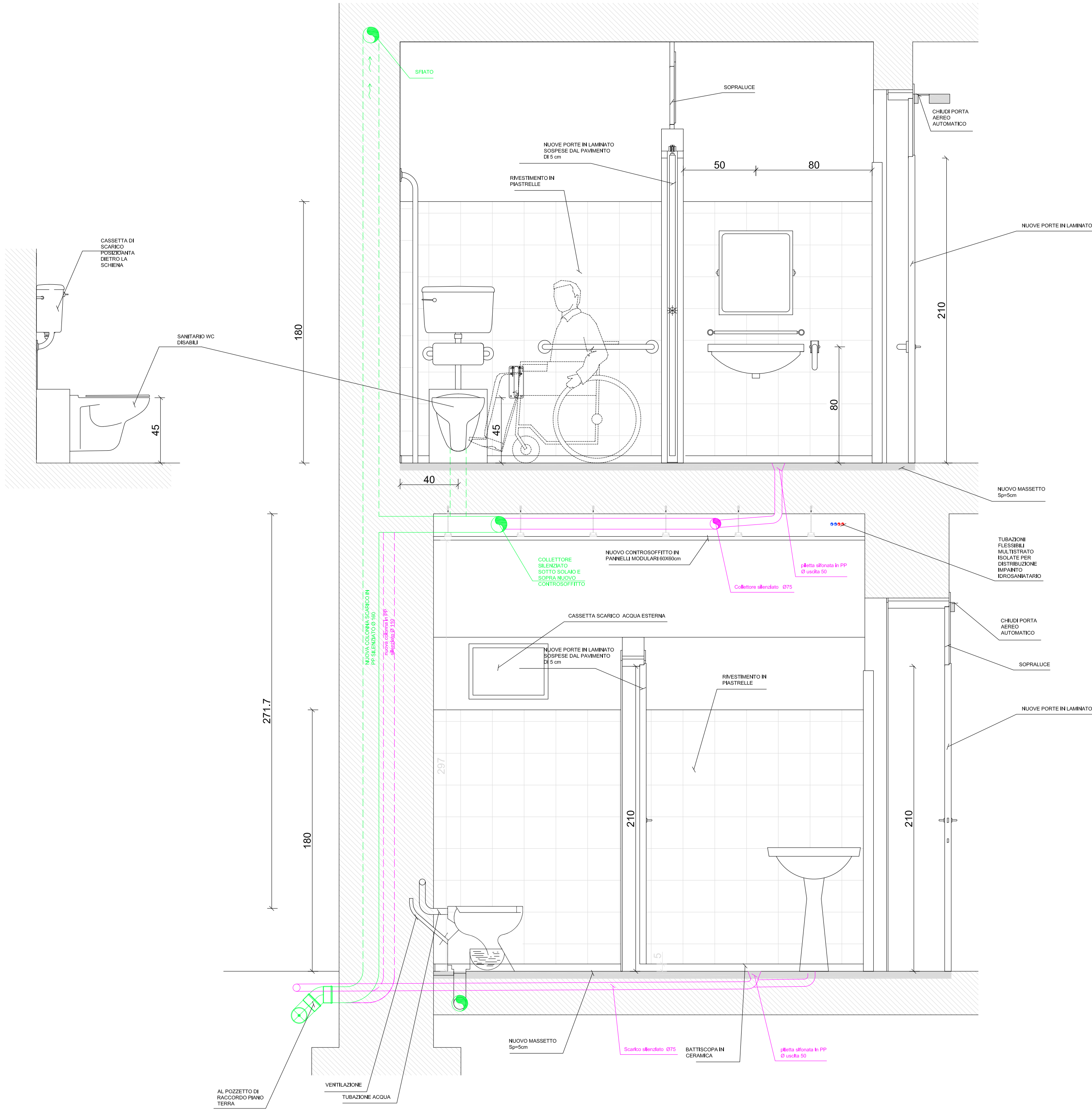
SEZIONE A-A DI PROGETTO SCALA 1:20
