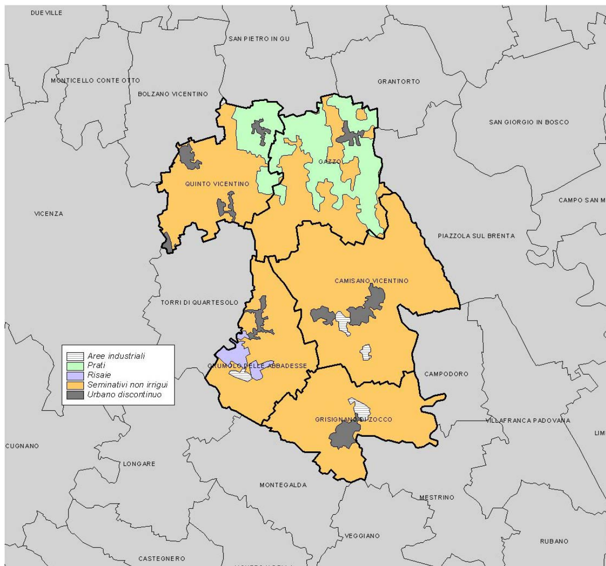
Fig. 2 – Calcolo di uso del suolo nell’ambito territoriale di riferimento- Fonte Corine Land Cover 1990
